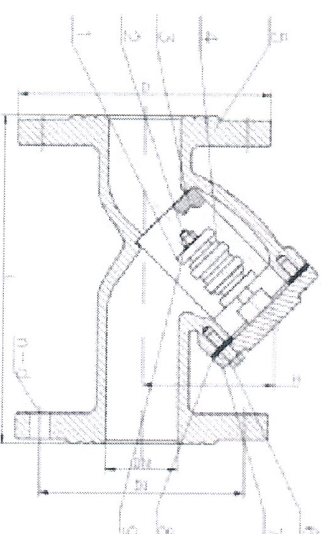
1 – шайба (углеродистая сталь, никелированная), 2 – стержень (нержавеющая сталь), 3 – сетка фильтрующая, 4 – магнит, 5 – корпус фильтра, 6 – болт, 7 – крышка фильтра, 8 – прокладка уплотнительная, 9 – гайка
