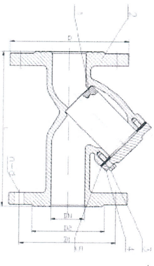
1 – сетка фильтрующая, 2 – корпус фильтра, 3 – болт, 4 – крышка фильтра, 5 – прокладка уплотнительная
