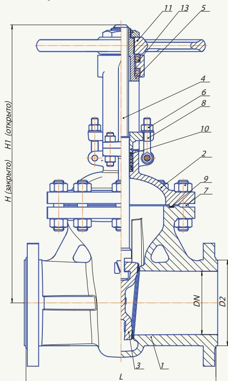
Задвижка, упругий клин, Ду 50 - 1200
