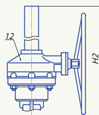
Задвижка с редуктором, Ду 300 - 1200
