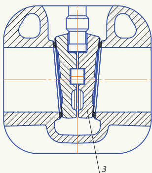
Задвижка, 2-х дисковый клин, Ду 80, 100
