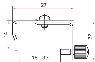
УПЗ-2 (нерж.)
