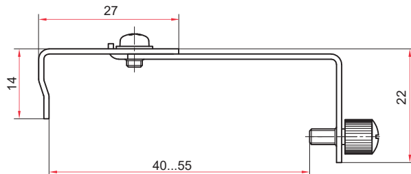
УПЗ-5 (нерж.)
