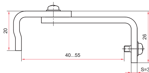
УПЗ-5 (АБС-пластик)
