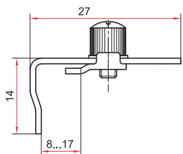
УПЗ-2 (нерж.)
